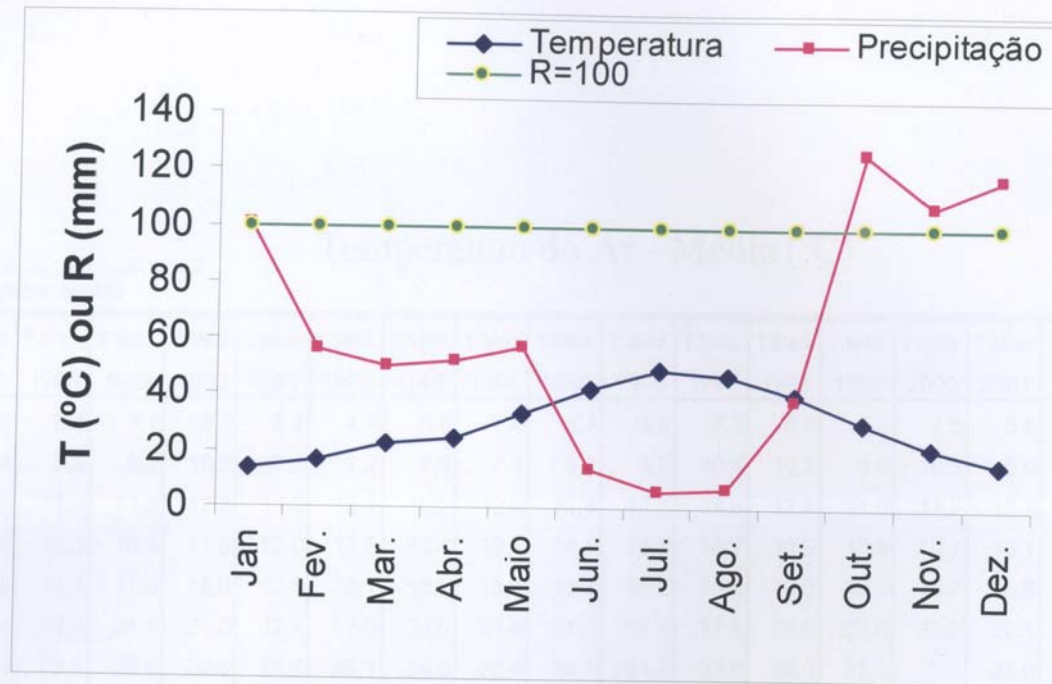
Figura 4- Diagrama Ombrotérmico para a região de Castelo Branco relativo ao período de 1986 -2005.
